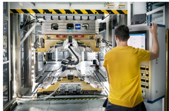
Hochdruckdosieranlage (links) und RTM-Versuchsstand (rechts, © Campus GmbH/ Moll) des AZL im Cluster Produktionstechnik auf dem RWTH Aachen Campus
